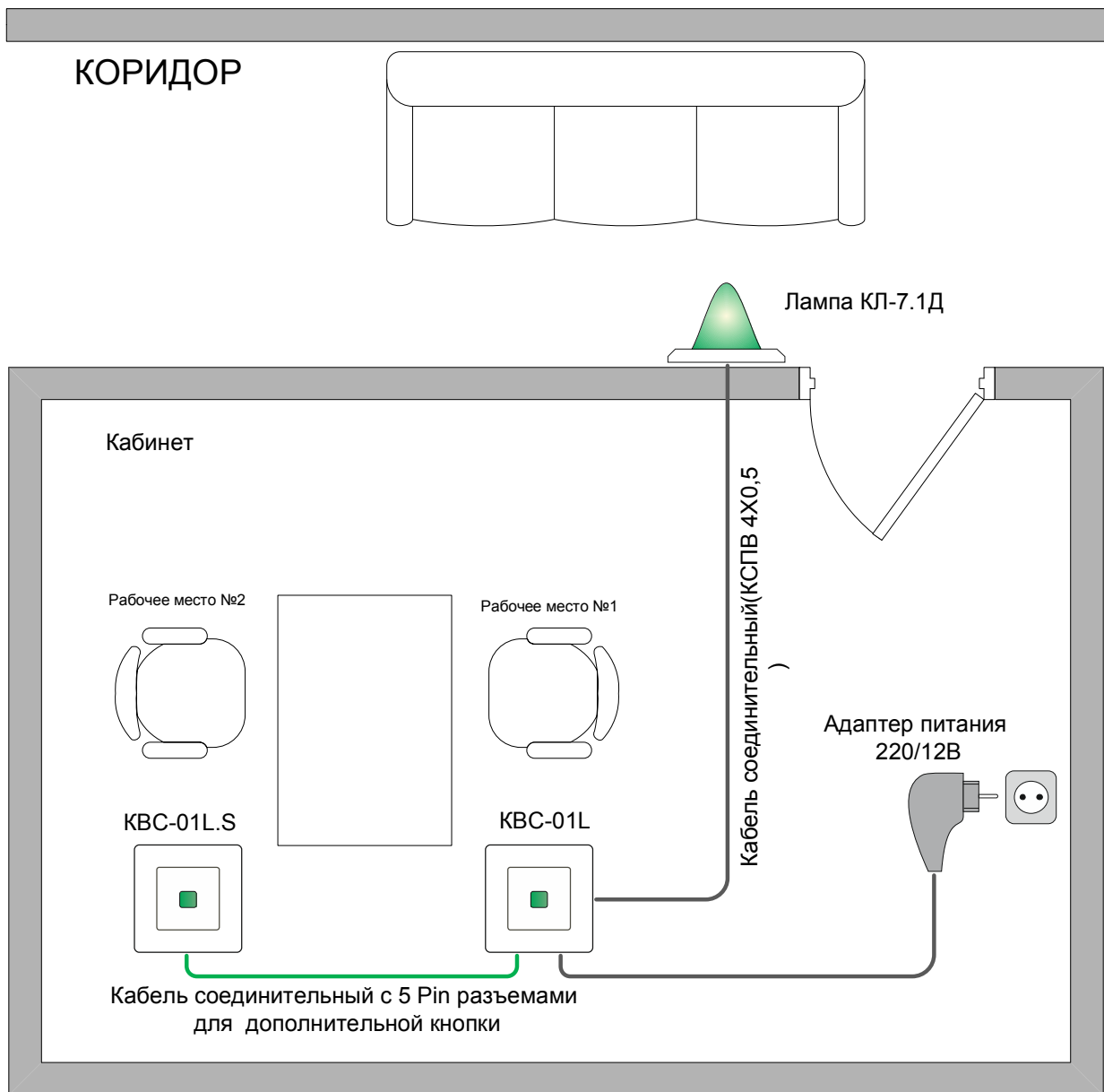
Рисунок 1. Схема структурная.
